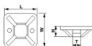
CASP
